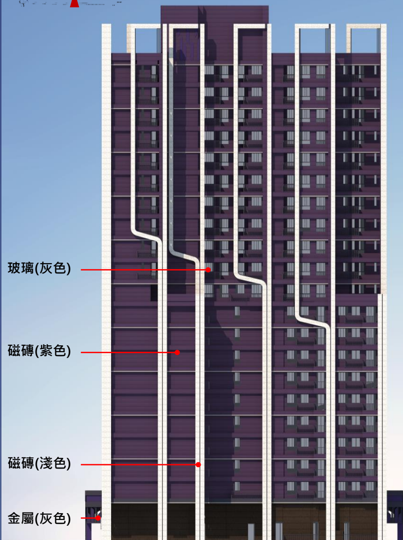
南向立面圖
