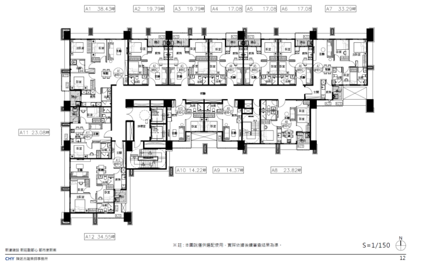
十三至十八層平面圖
