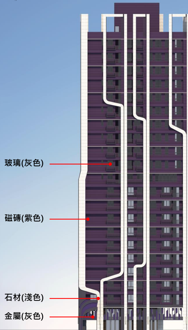
西向立面圖
